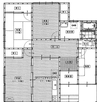
町営住宅平面図 天神団地Aタイプ
