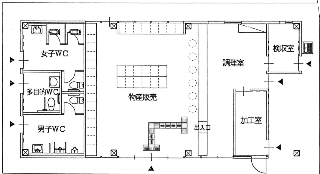
井川町農産物直売・食材供給施設平面図
