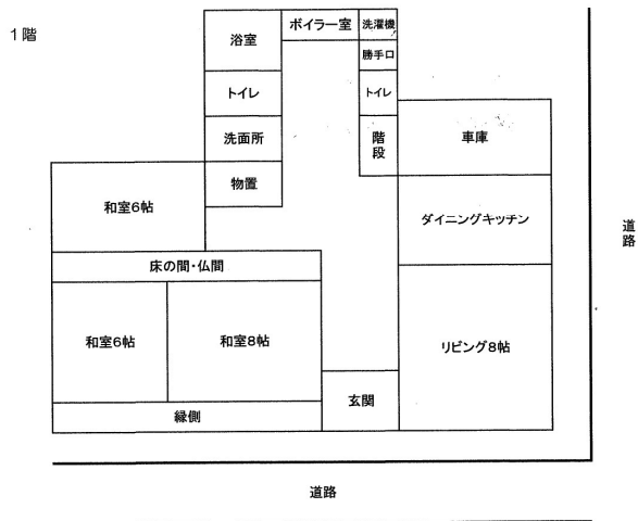
井川町北川尻字海老沢樋ノ口97番地17 建物間取図
